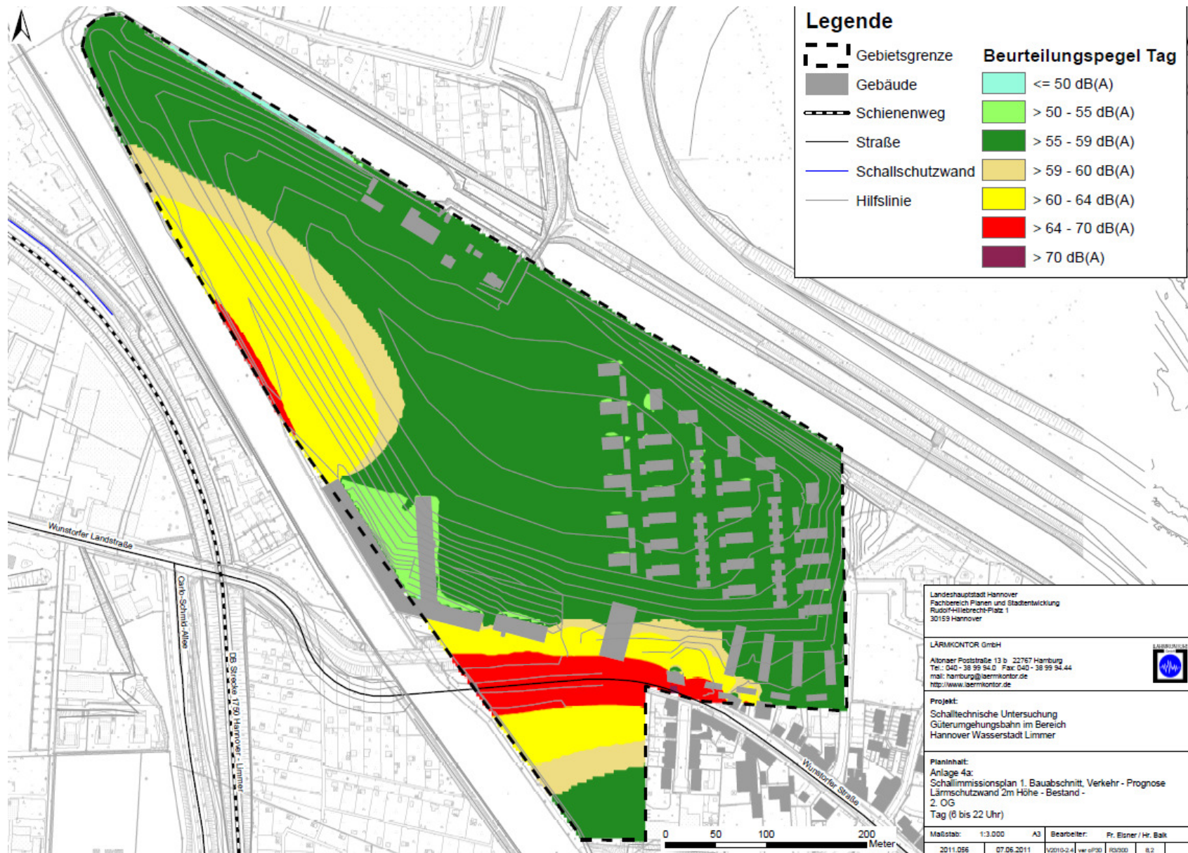
Schallimmissionsplan 1. Bauabschnitt Verkehr – Prognose Lärmschutzwand 2 m Höhe – Bestand / 2. OG Tag (6 bis 22 Uhr)
